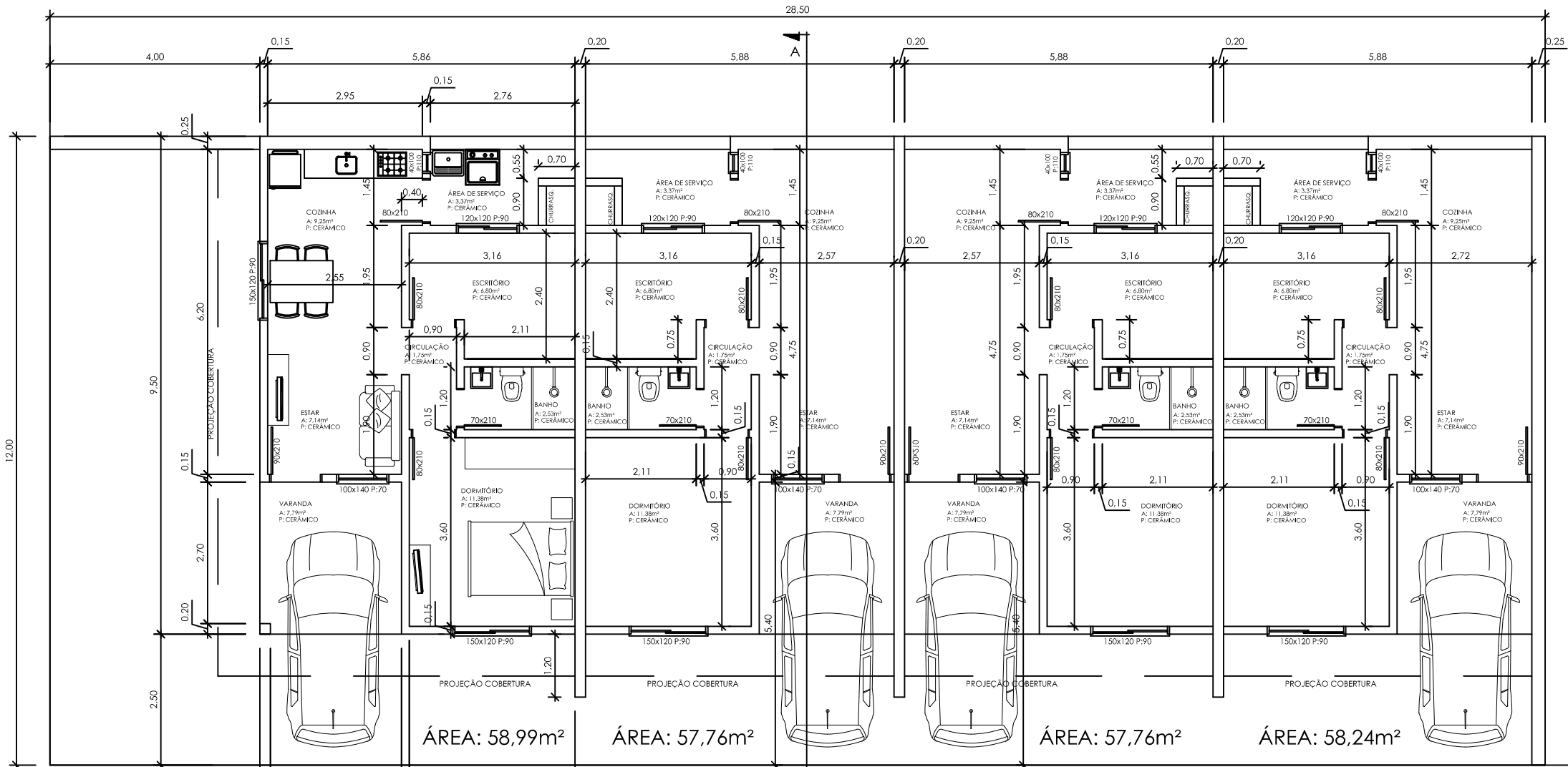
PLANTA BAIXA ÁREA: 232,75m 2 ESCALA: 1/50
